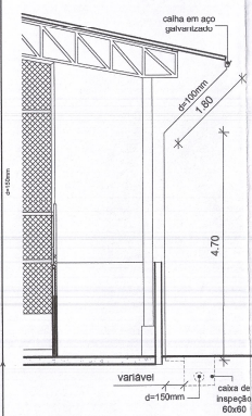
2 Tubo de Queda - Calha 1 : 50
