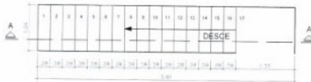
PLANTA BAIXA ESCADA ESC 1/25
